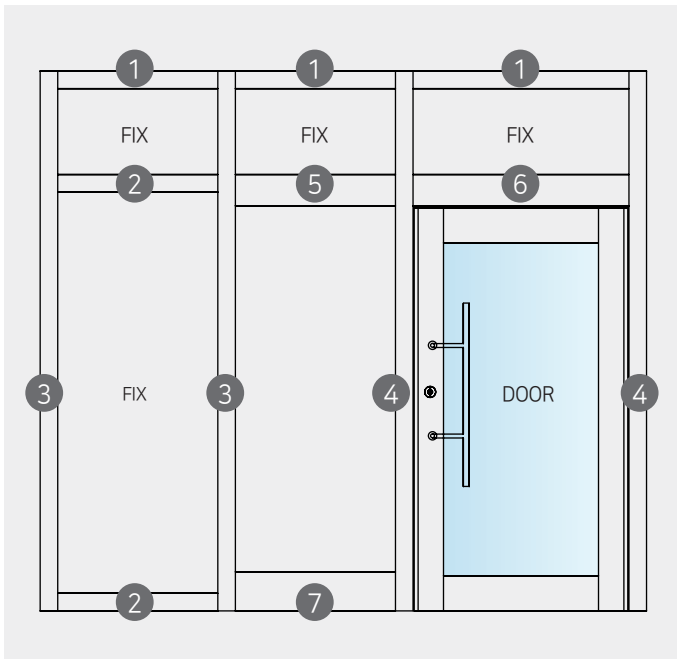
단열프레임 형재 기호 적용표 (예)
