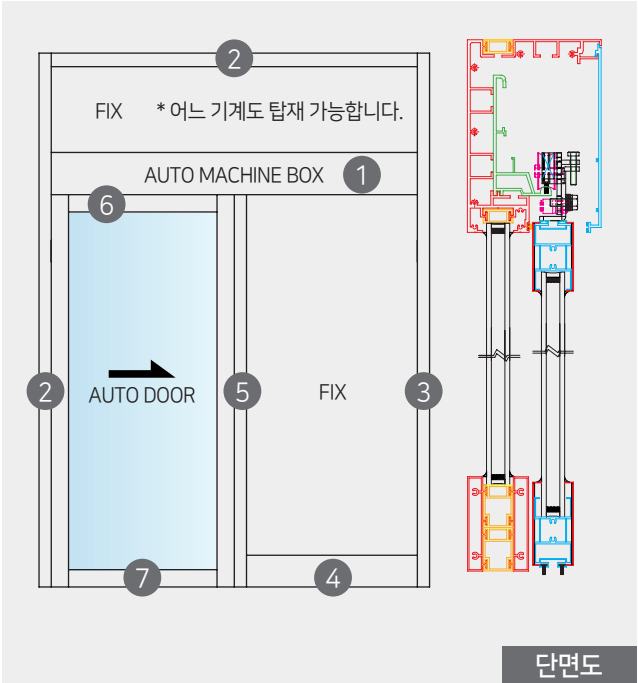
프레임 기호 적용표 (예)
