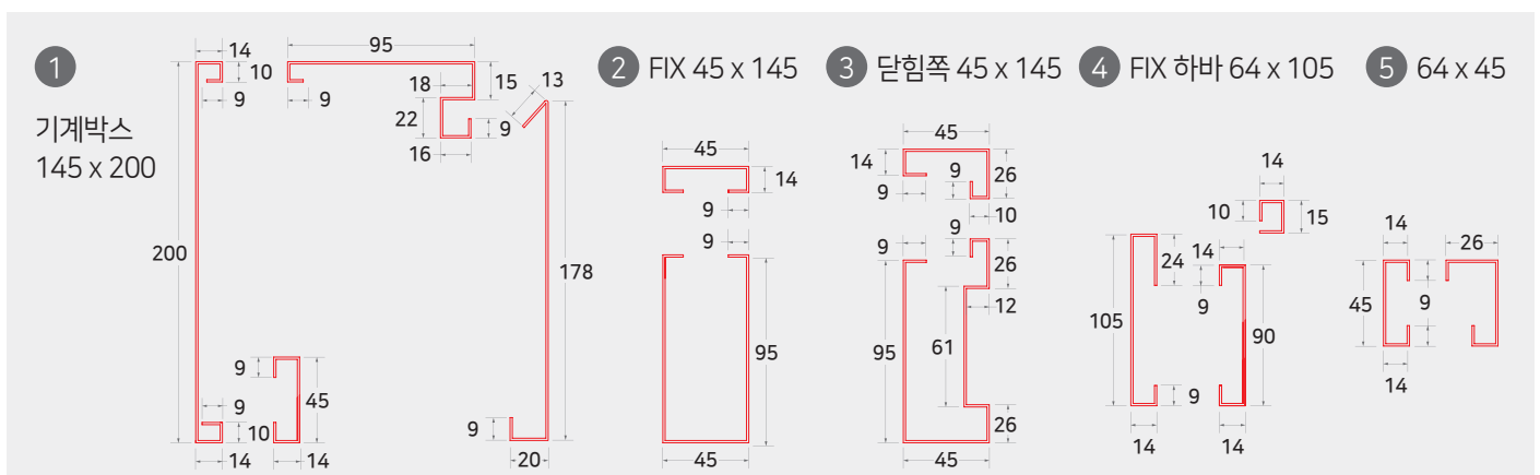
스텐레스 프레임 절곡도
