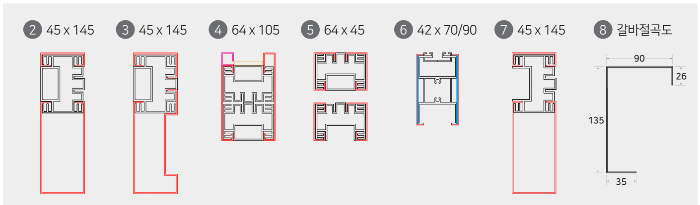
단열 스텐레스 프레임 조립도
