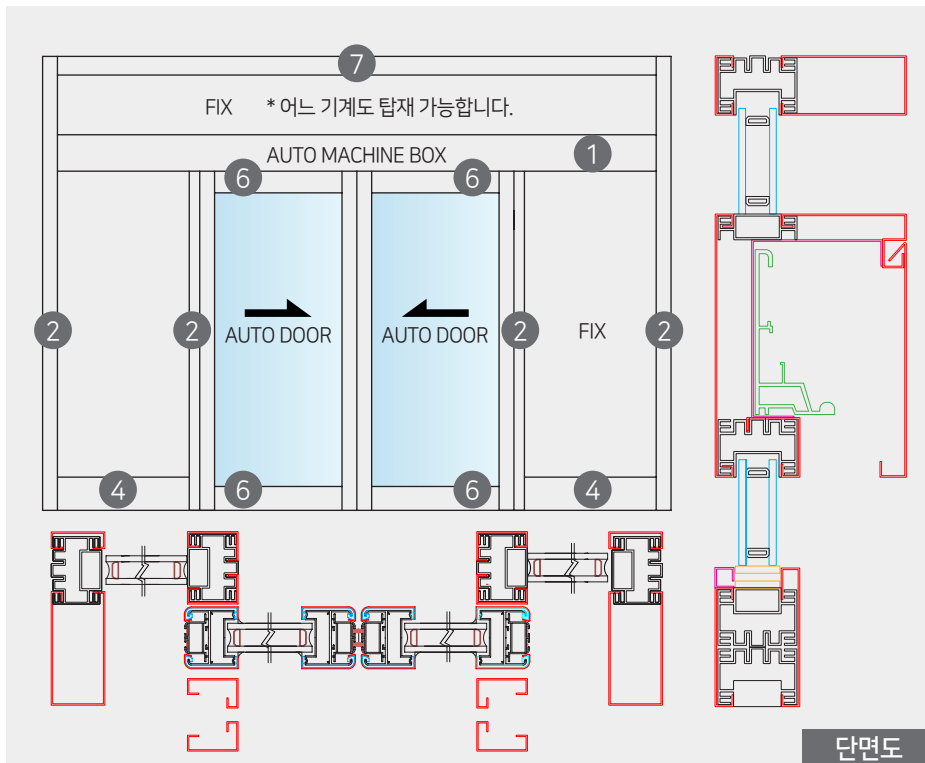
스텐레스 프레임 단열재 기호 적용표 (예)
